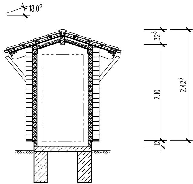
SCHNITT A-A
