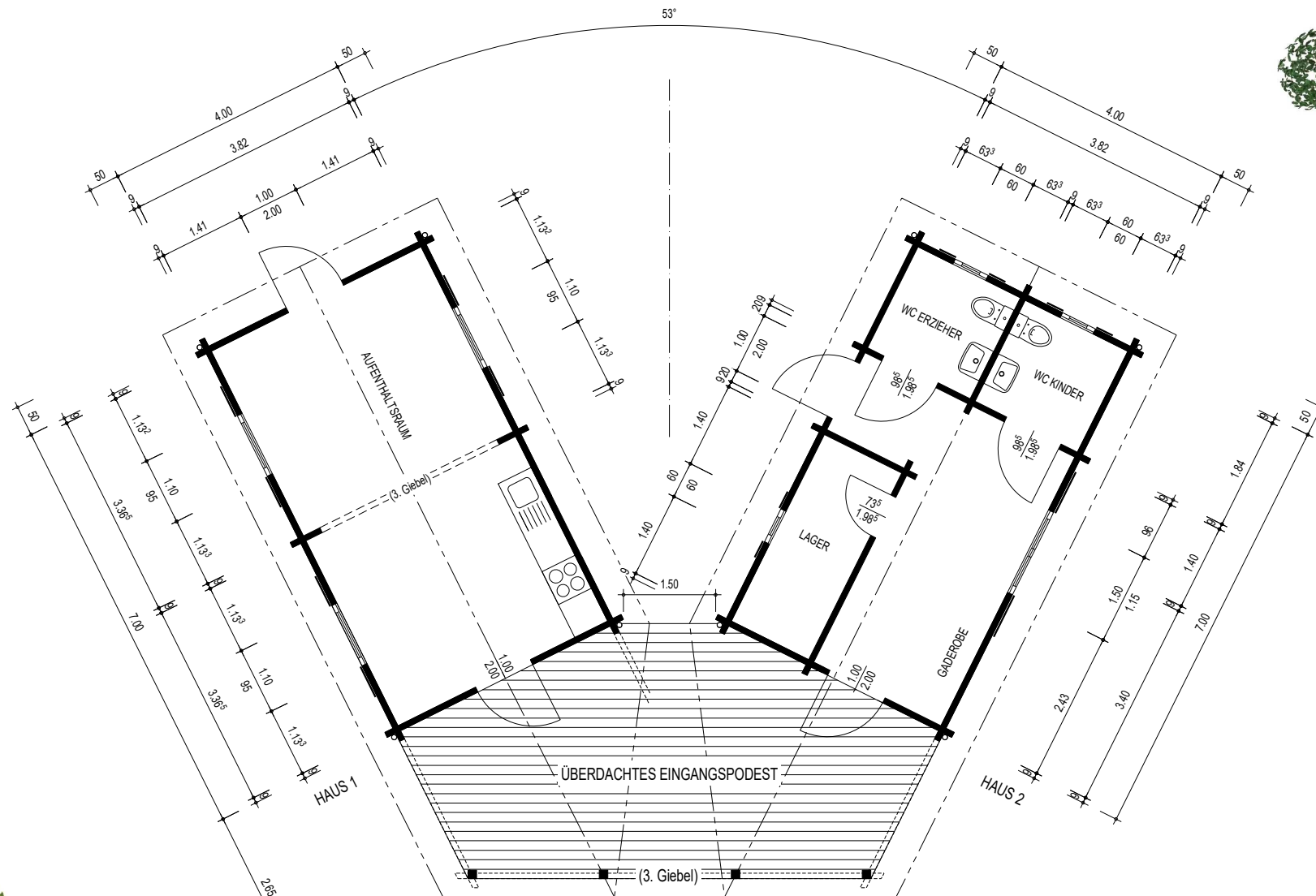
GRUNDRISS Maßstab: 1:100
